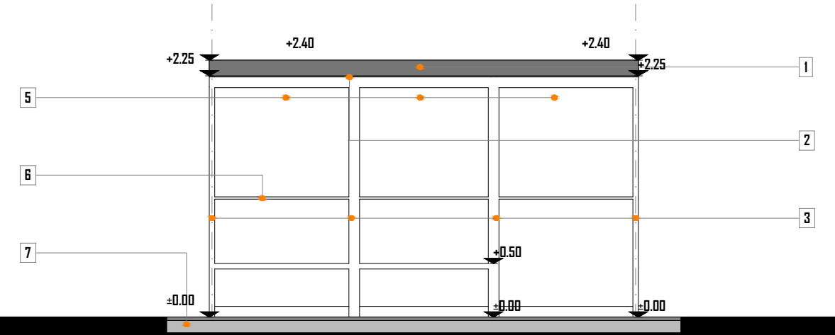
FATADA POSTERIOARA
